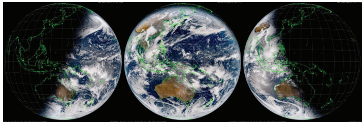
2023年12月21日の全球トゥルーカラー再現画像(出典:気象庁)
